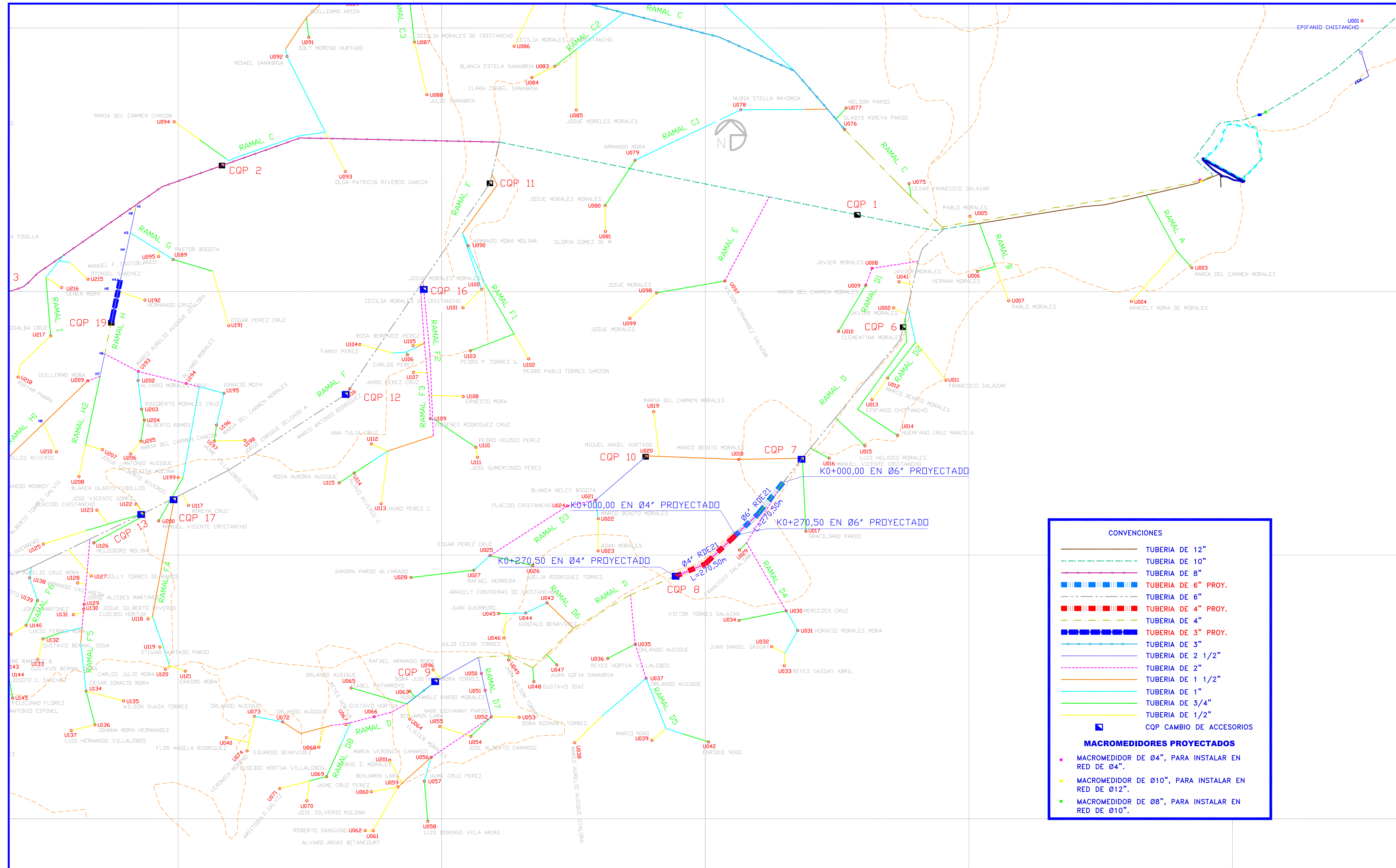
PLANTA RAMAL D Y LOCALIZACIÓN DE MACROMEDIDORES ESCALA 1:7.500
