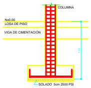
DETALLE GENERAL ZAPATA ESC. 1:20
