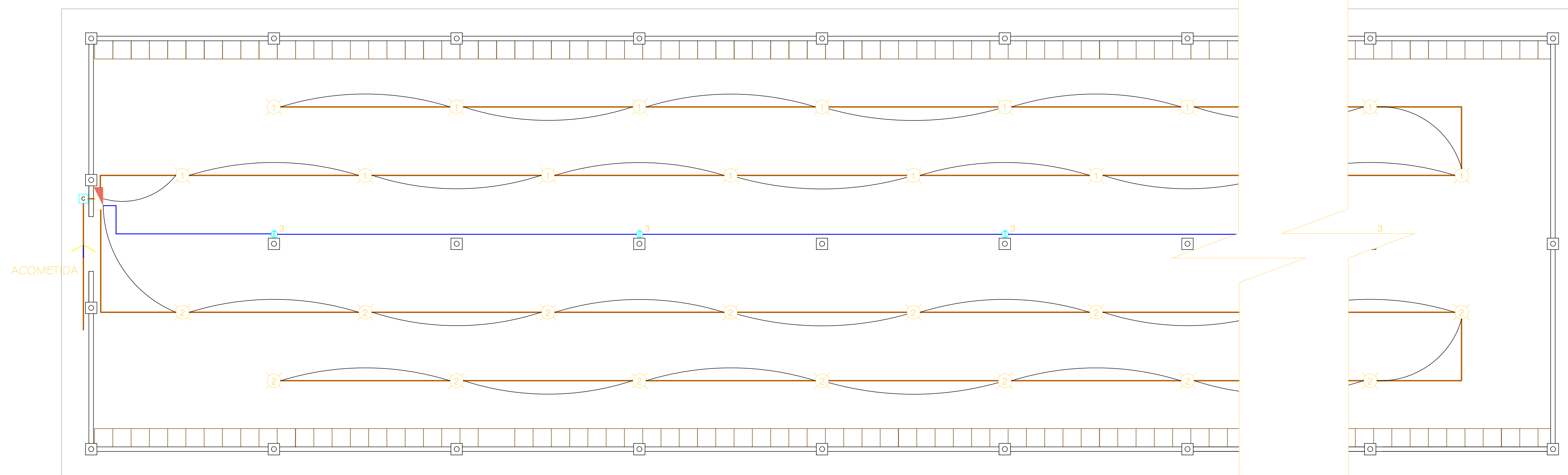
PLANTA INSTALACION ELECTRICA ESCALA : 1 : 75
