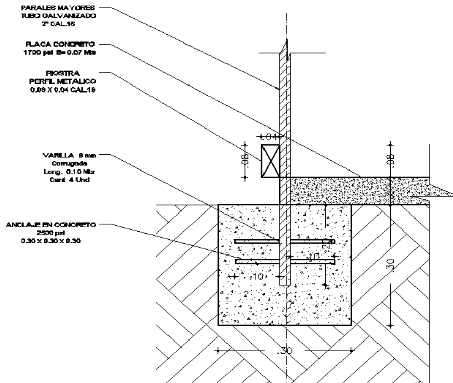
PLANO No.3 – DETALLE DE ANCLAJE PARALES MAYORES Y MENORES ÍTEM 2 Y 4
