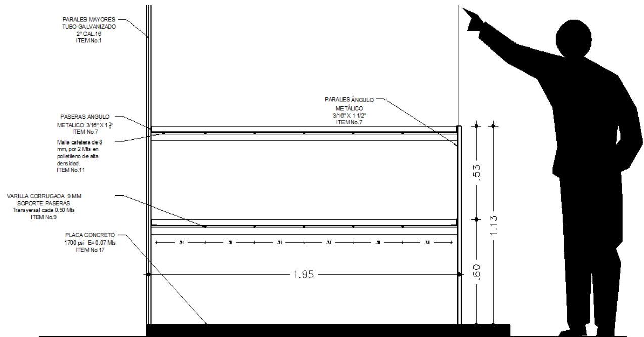
PLANO No.7 – DETALLE FACHADA PASERA
