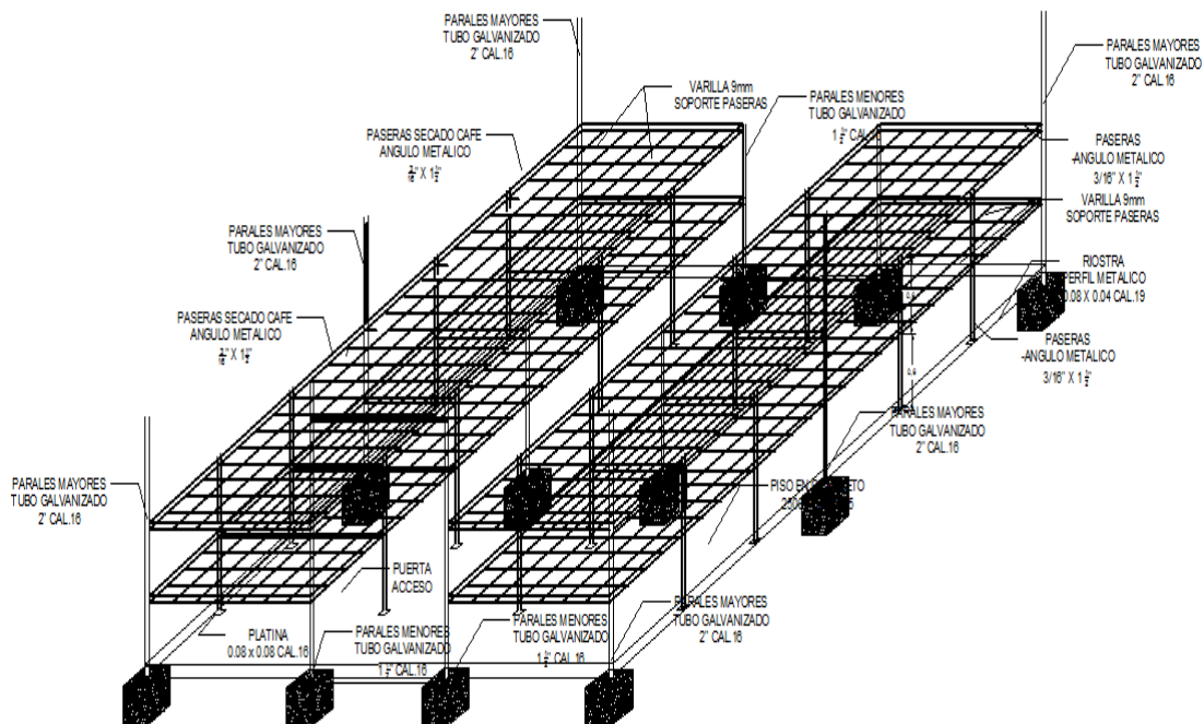
PLANO No.6 – PLANTA ESTRUCTURA DE PASERAS DE SECADO
