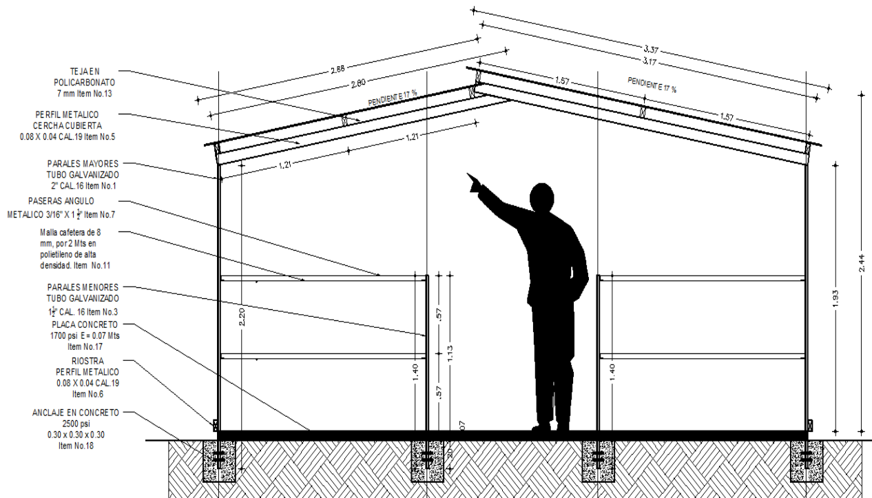
PLANO No.5 – CORTE TRANSVERSAL
