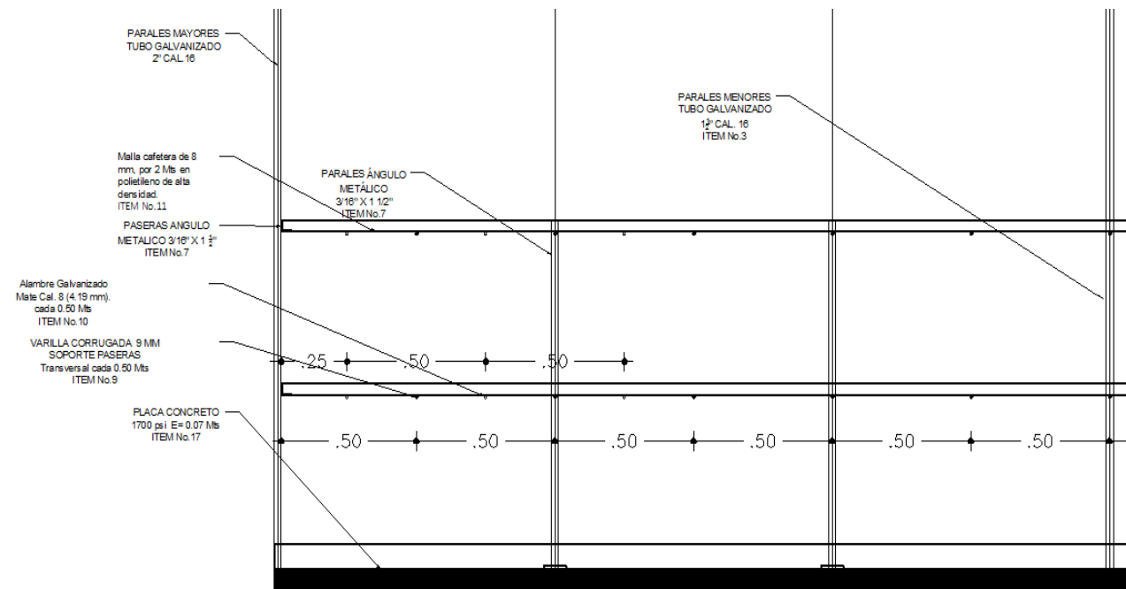
PLANO No.8 – PLANO LATERAL SECCIÓN PASERA
