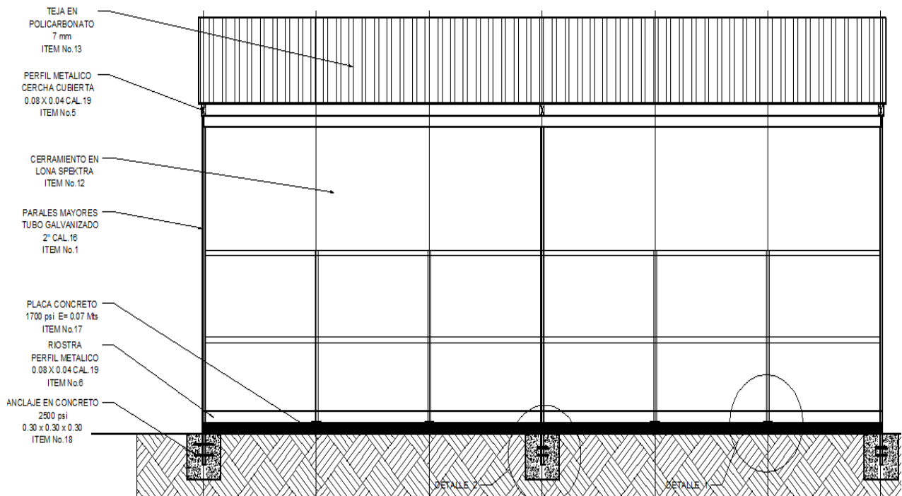
PLANO No.4 – PERFIL LATERAL
