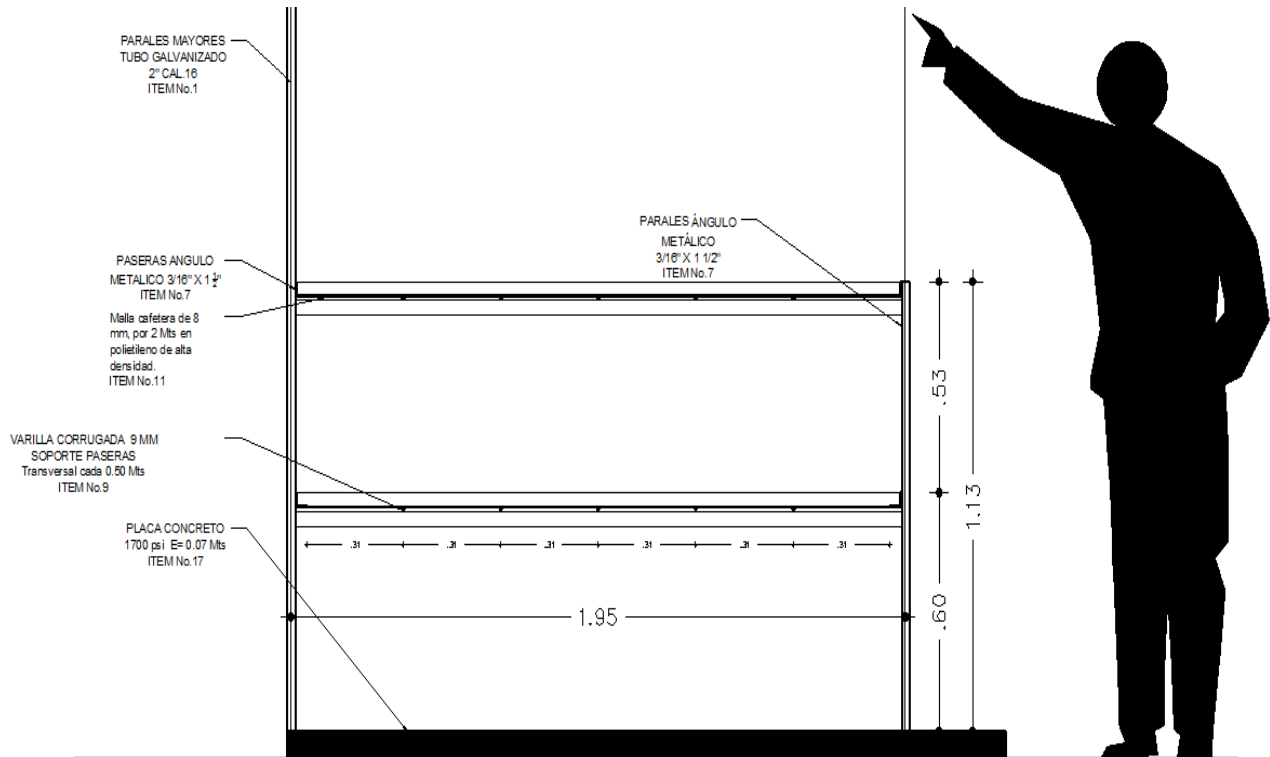
PLANO No.7 – DETALLE FACHADA PASERA
