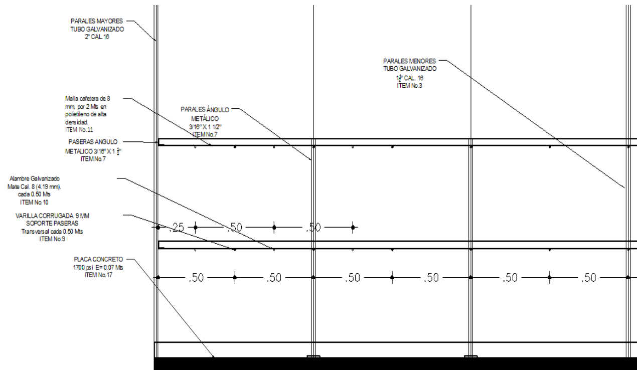
PLANO No.8 – PLANO LATERAL SECCIÓN PASERA
