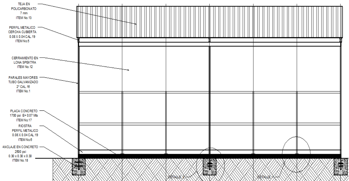
PLANO No.4 – PERFIL LATERAL
