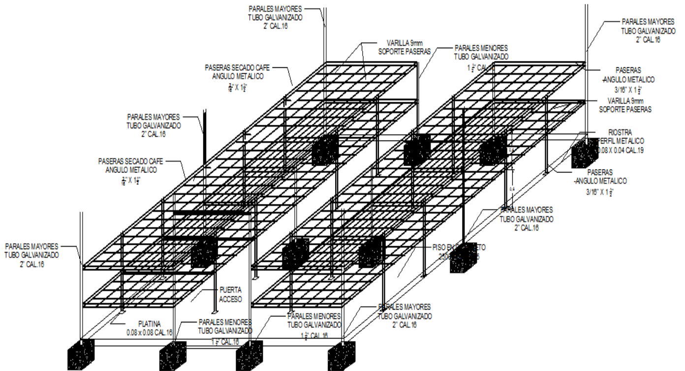
PLANO No.6 – PLANTA ESTRUCTURA DE PASERAS DE SECADO
