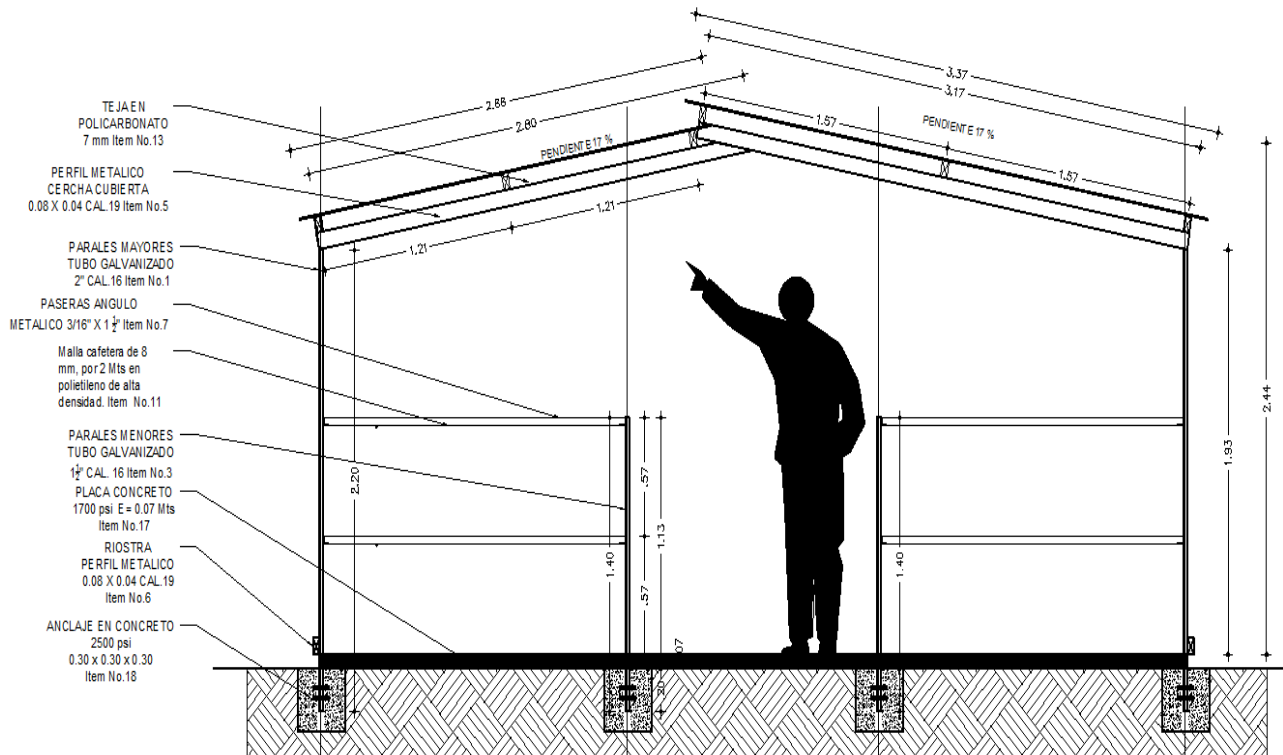
PLANO No.5 – CORTE TRANSVERSAL
