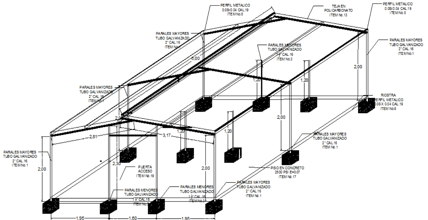
PLANO No.2 – PLANTA ESTRUCTURAL
