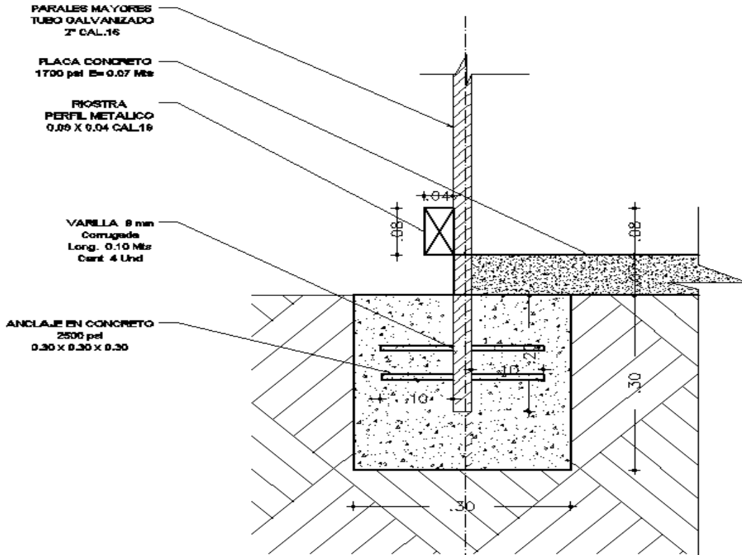
PLANO No.3 – DETALLE DE ANCLAJE PARALES MAYORES Y MENORES ITEM 2 Y 4
