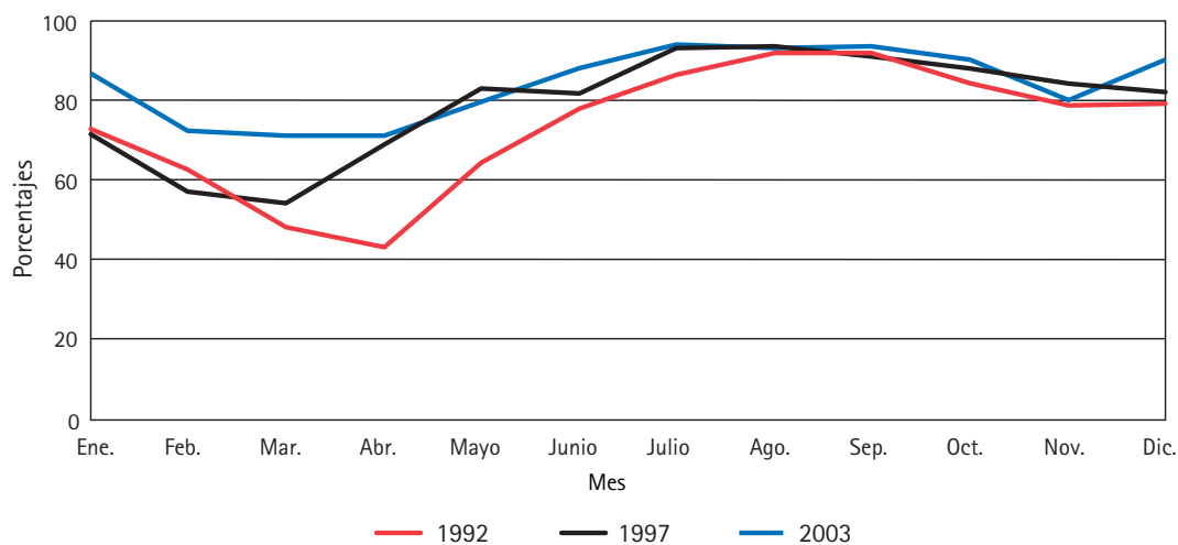
Figura I. Efectos de la reforestación sobre la humedad relativa, años 1992-2003
