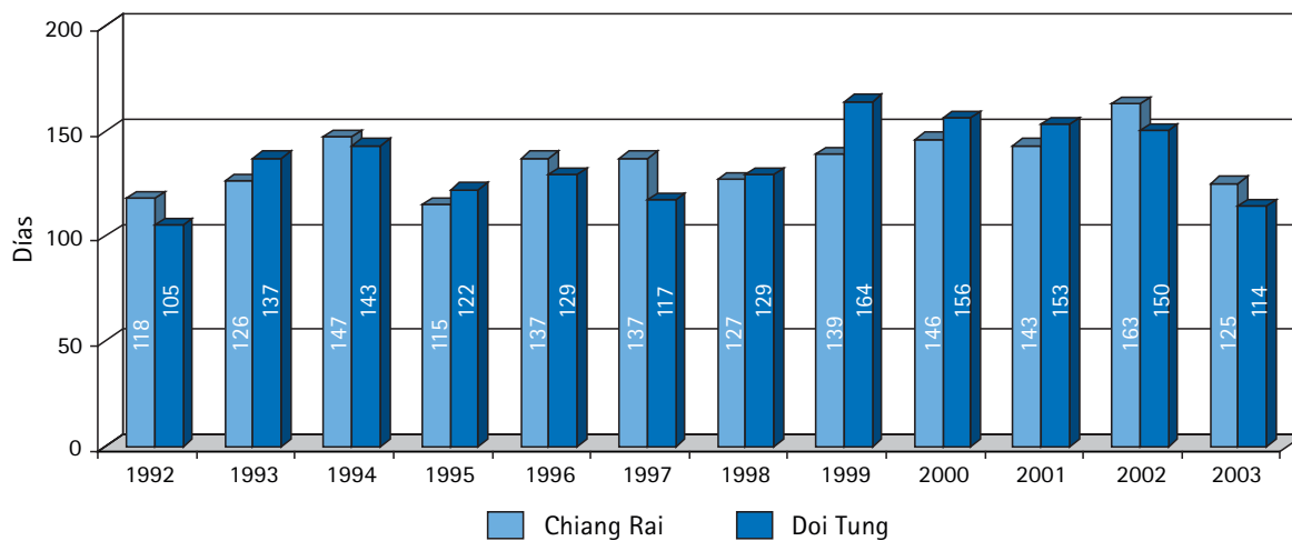
Figura V, Efectos de la reforestación sobre la distribución de las precipitaciones anuales, 1992-2003
