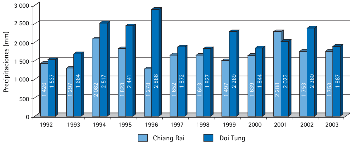
Figura IV. Efectos de la reforestación sobre las precipitaciones anuales, 1992-2003
