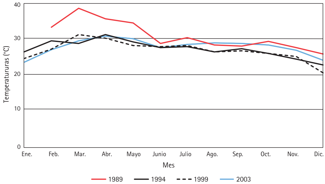
Figura III. Efectos de la reforestación sobre las temperaturas máximas, 1989-2003
