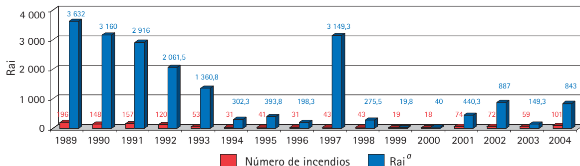
Figura VI. Incidencia de los incendios forestales, 1989-2004
